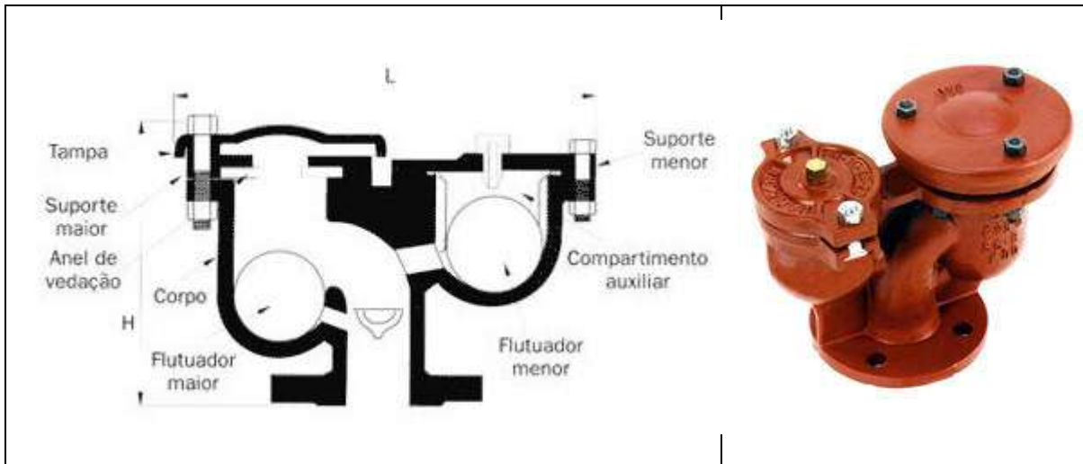
Figura 12.2 - Ventosa Tríplice Função
